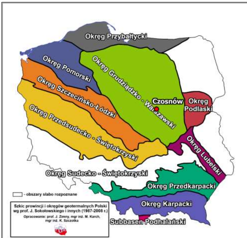
Rysunek 6. Położenie gminy Czosnów na tle okęgów geotermalnych Polski
